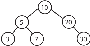
Не является законченным бинарным деревом
