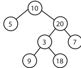
Полное бинарное дерево
