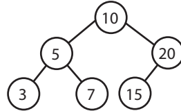
Законченное бинарное дерево
