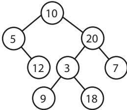
Не является полным бинарным деревом
